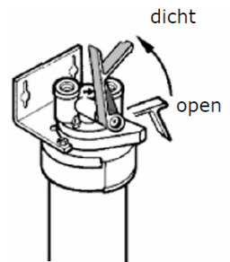
Fig 2. Filterkop
